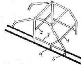
Zeichnung 20
