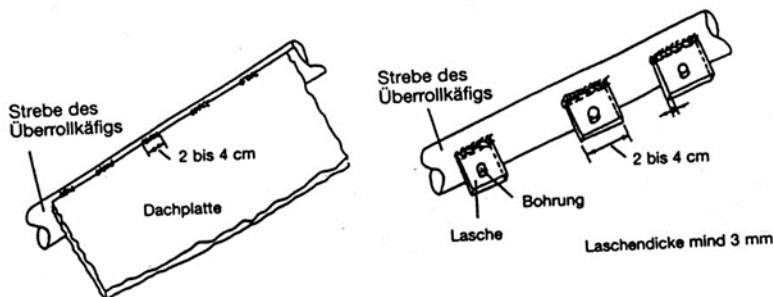
Zeichnung 6 (Dach)
